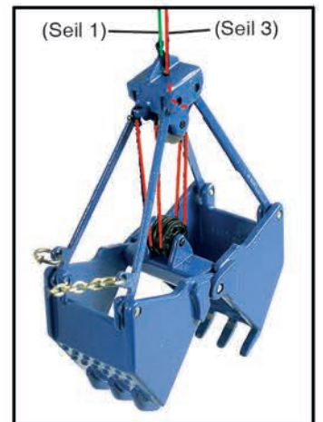
05. die Greifer-Seile (1) und (3) am Greifer befestigen bzw. aufseilen
