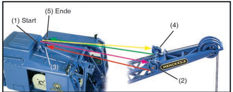
04. das Gittermast-Halteseil (2) aufseilen
